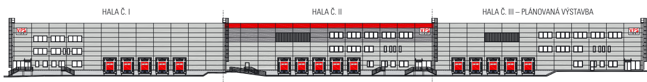
VÝCHODNÍ POHLED
